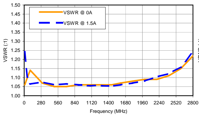
RF VSWR
