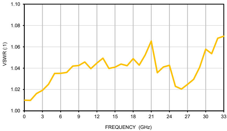
2.92-MALE VSWR
