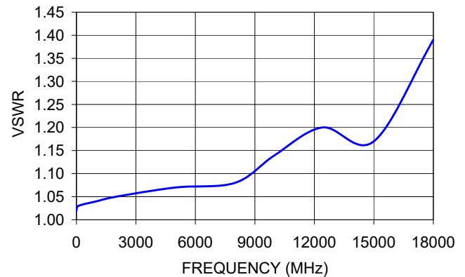
BW-S6W2+ VSWR
