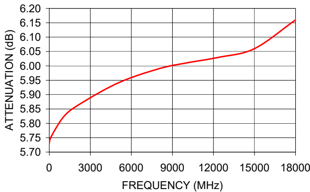
BW-S6W2+ ATTENUATION
