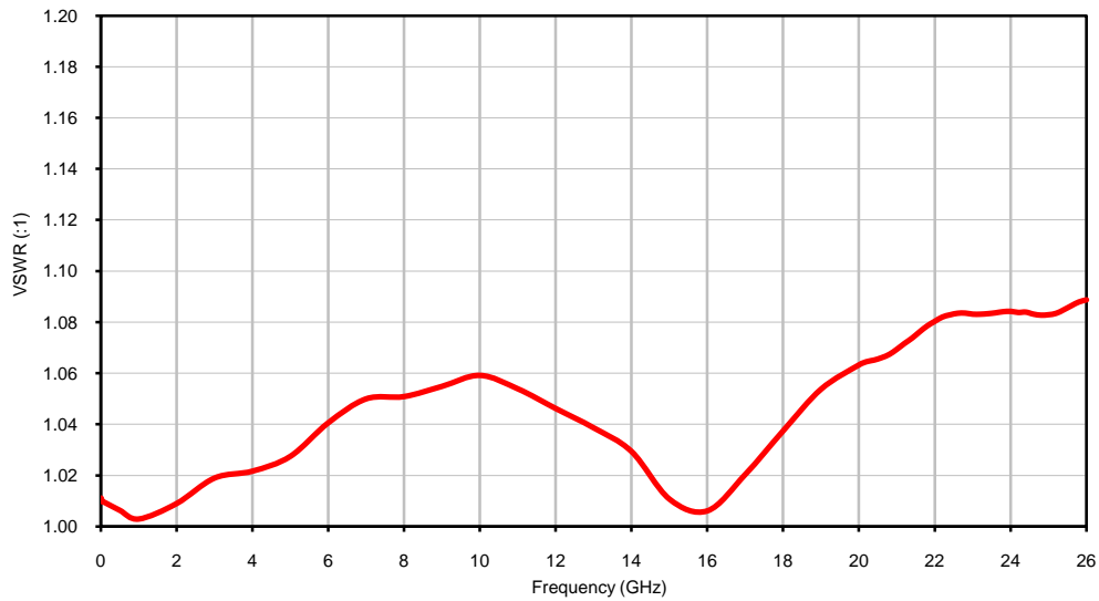
VSWR
