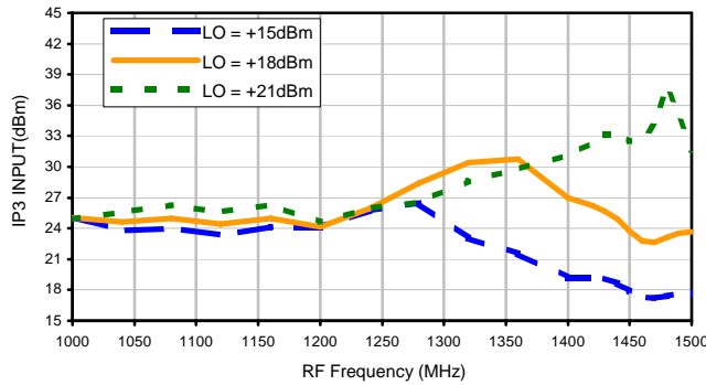
IP3 INPUT
