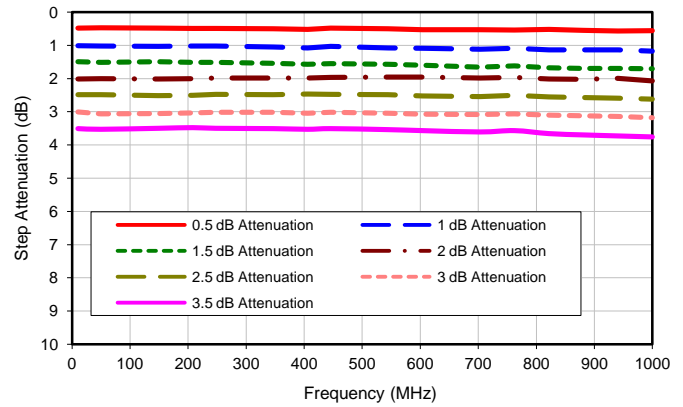
Step Attenuation
