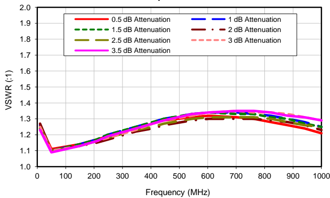
Input VSWR
