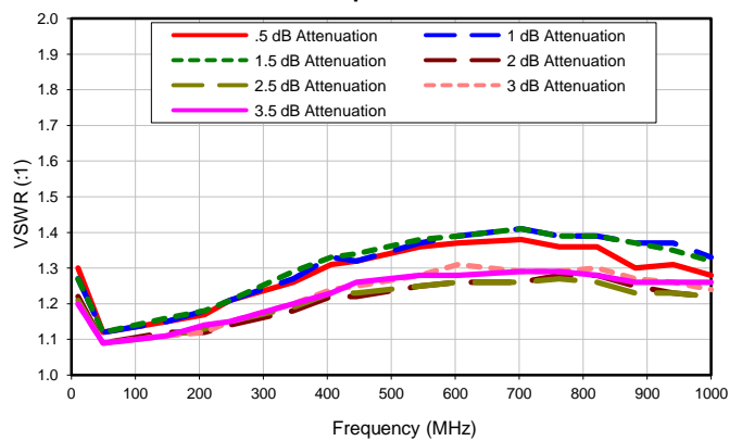
Output VSWR
