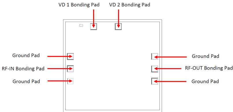
Fig 2. Die Layout
