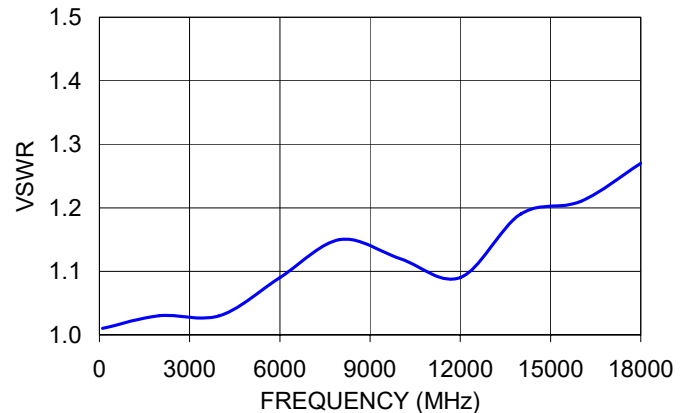
BW-N1W5+ VSWR
