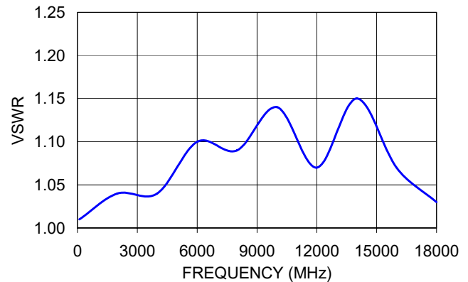
BW-N3W5+ VSWR
