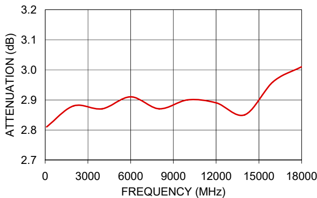
BW-N3W5+ ATTENUATION
