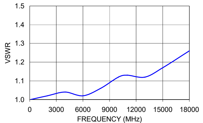
BW-N5W5+ VSWR
