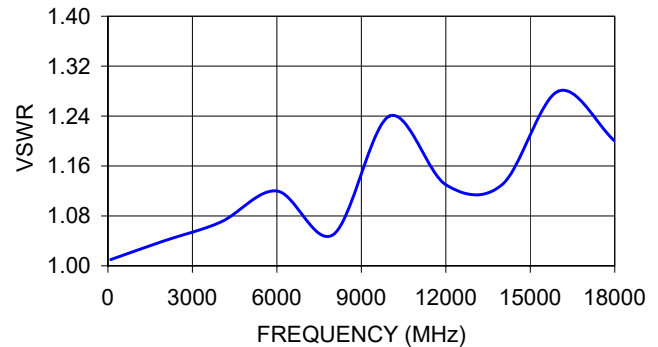
BW-S10W5+ VSWR
