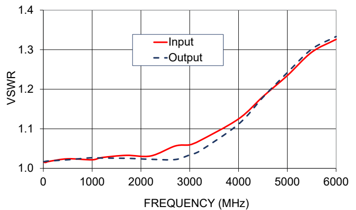
EQY-2-63+ VSWR
