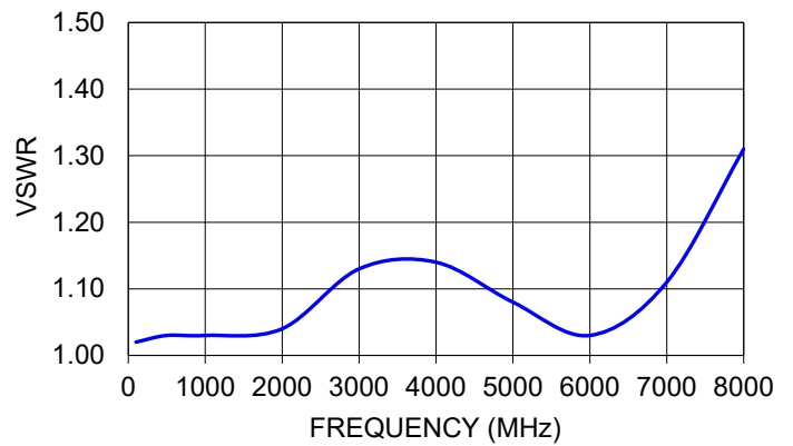
GAT-2+ VSWR
