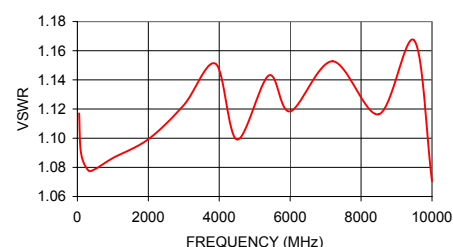
VSWR
