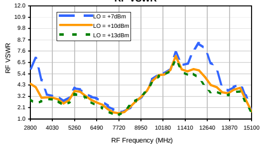
RF VSWR
