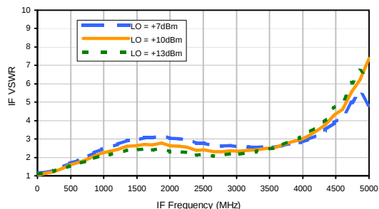
IF VSWR
