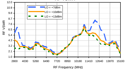
RF VSWR
