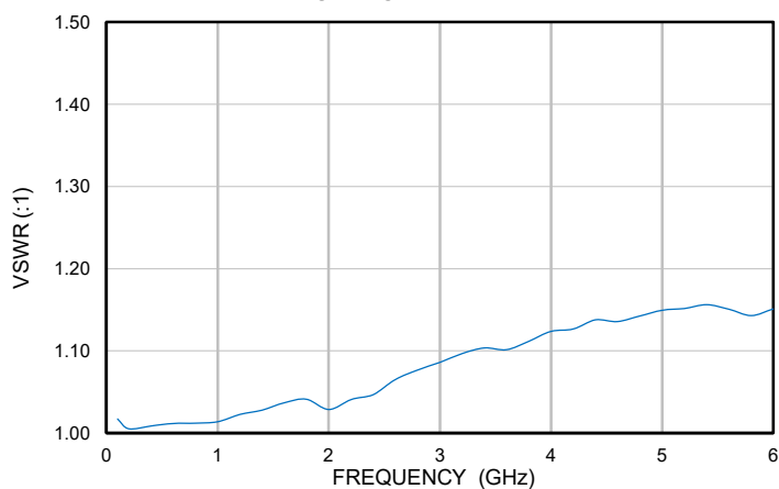
Right Angle SMA VSWR (+25°C)
