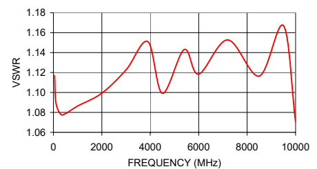
ADCH-80+ VSWR
