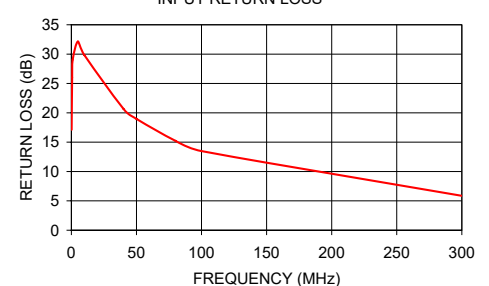
ADTT1.5-1 INPUT RETURN LOSS
