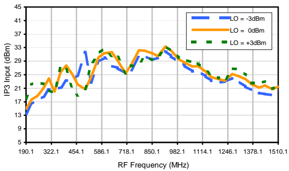
IP3 Input
