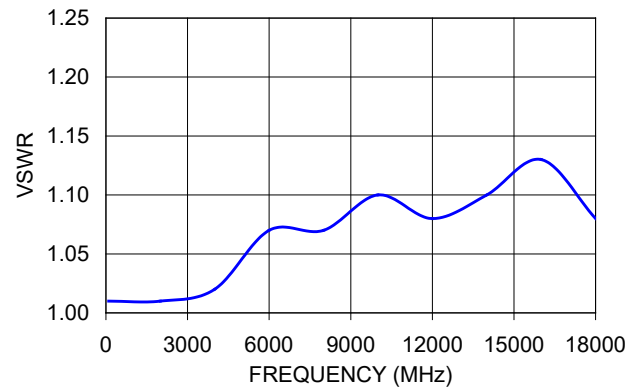
BW-N15W5+ VSWR
