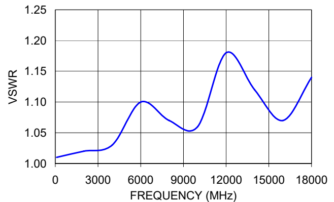
BW-N8W5 VSWR
