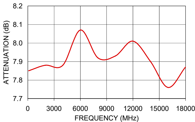
BW-N8W5 ATTENUATION
