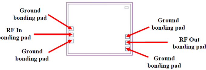
Fig 1. Die Layout
