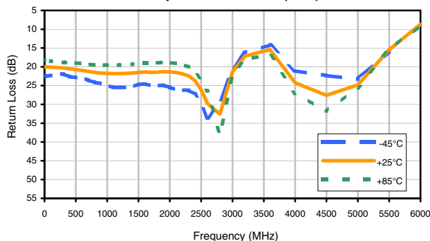
Input Return Loss (4dB)
