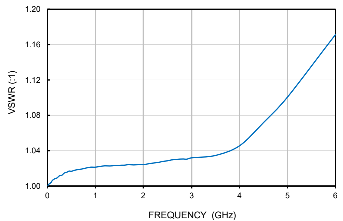
DIN FEMALE VSWR (+25 °C)
