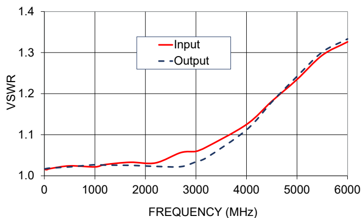
EQY-2-63+ VSWR
