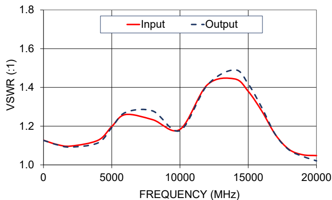
EQY-5-24+ VSWR
