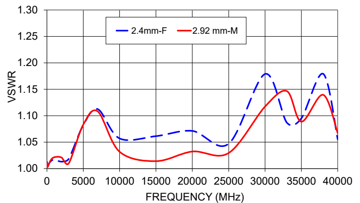
KMR-24F+ VSWR
