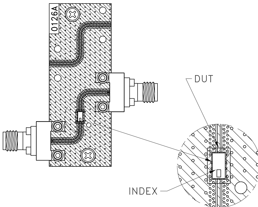
TB-LFCN-2352C+
