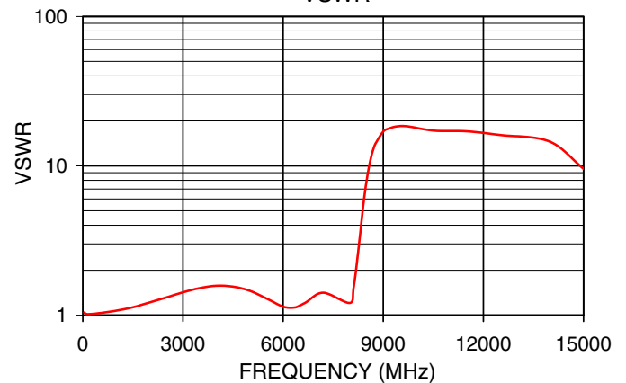
LFCN-7200+ VSWR
