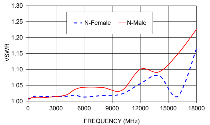
NF-NMR50-18+ VSWR
