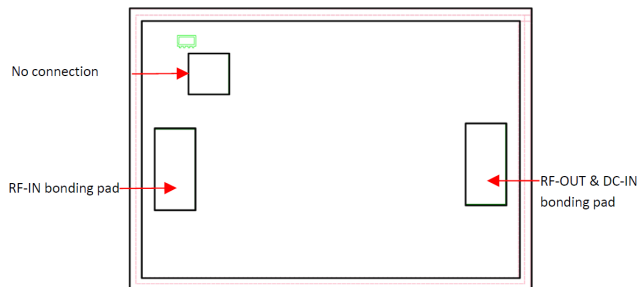
Fig 2. Die Layout
