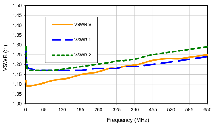
VSWR
