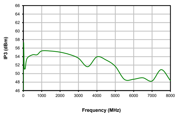
IP3 @ 0dB Attenuation
