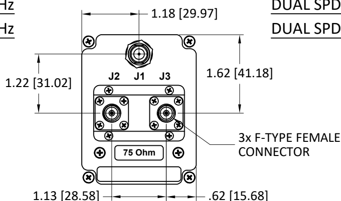
SPDT 2.15GHz
