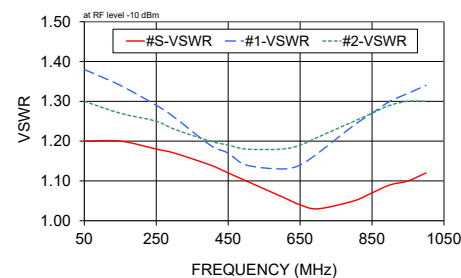
VSWR
