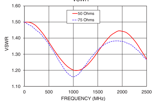
SFMP-5075+ VSWR
