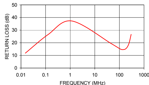
T1-6T INPUT RETURN LOSS
