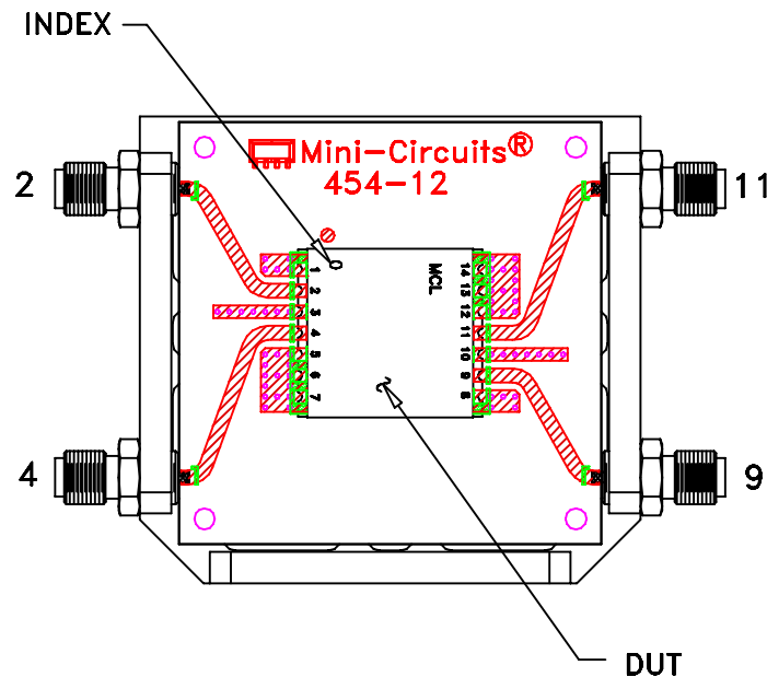
TB-516+
