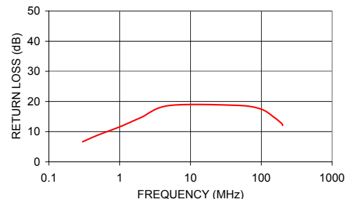
TMO-6-1+ INPUT RETURN LOSS
