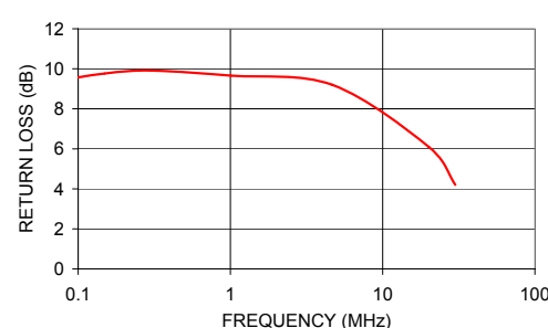
TTMO-25-1+ INPUT RETURN LOSS
