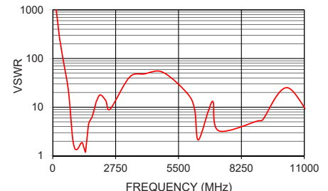
VBFZ-1065-S+ VSWR
