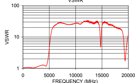
VLF - 3800+ VSWR
