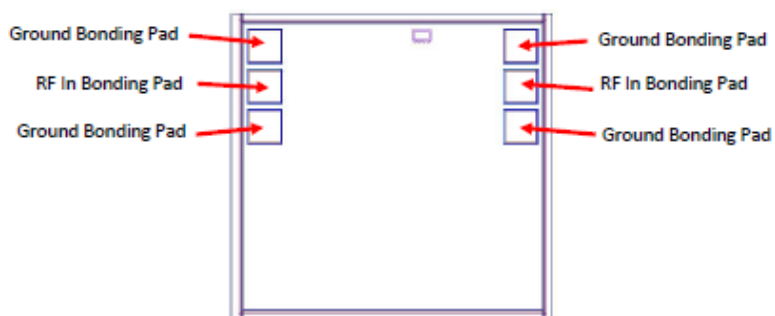
Fig 2. Die Layout
