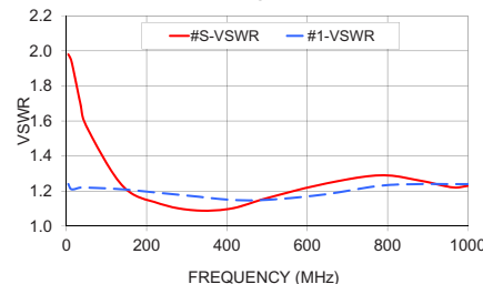
ZFSC-8-4-75+ VSWR
