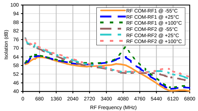
Isolation @ VDD=+5V over Temperature RF COM-RF1 & RF COM-RF2
