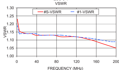
ZSC-3-1 VSWR
