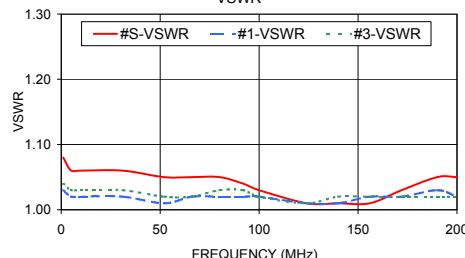
ZSC-4-1-75+ VSWR
