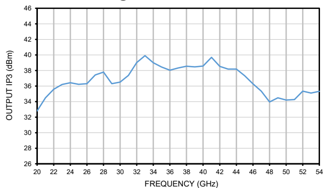
OIP3 @MINIMUM ATTENUATION
