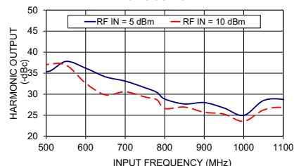
ZX90-2-11-S+ HARMONIC OUTPUT F1
